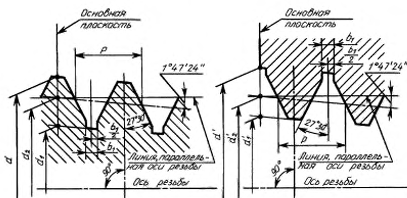
Профиль резьбы калибра-кольца
