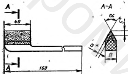
Черт. 5 Тип 06
