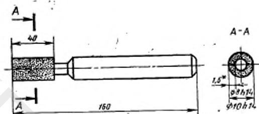
Черт. 4 Тип 05
