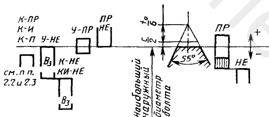
Калибры для контроля болтов (наружной резьбы)
