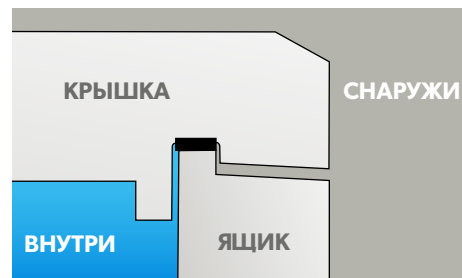
Лабиринтное уплотнение предотвращает проникновение тепла внутрь.
